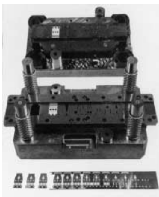
Matriz progresiva fabricada con SVERKER 21 para la producción de series largas de una complicada pieza troquelada.
